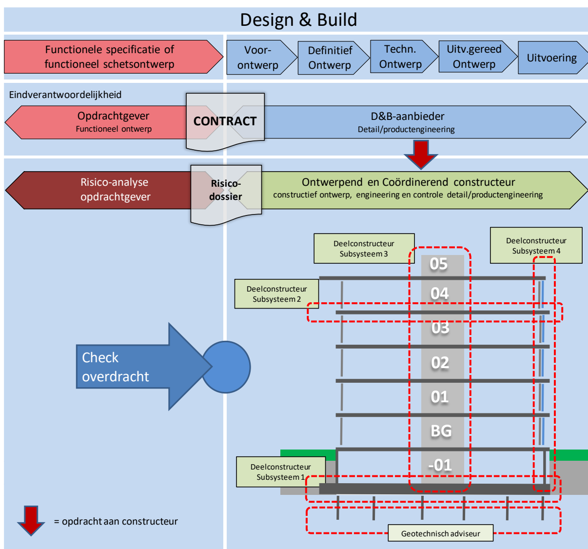
Figuur 9: contracteren van constructeurs bij Design & Build (Bron: BAM Advies & Engineering)
